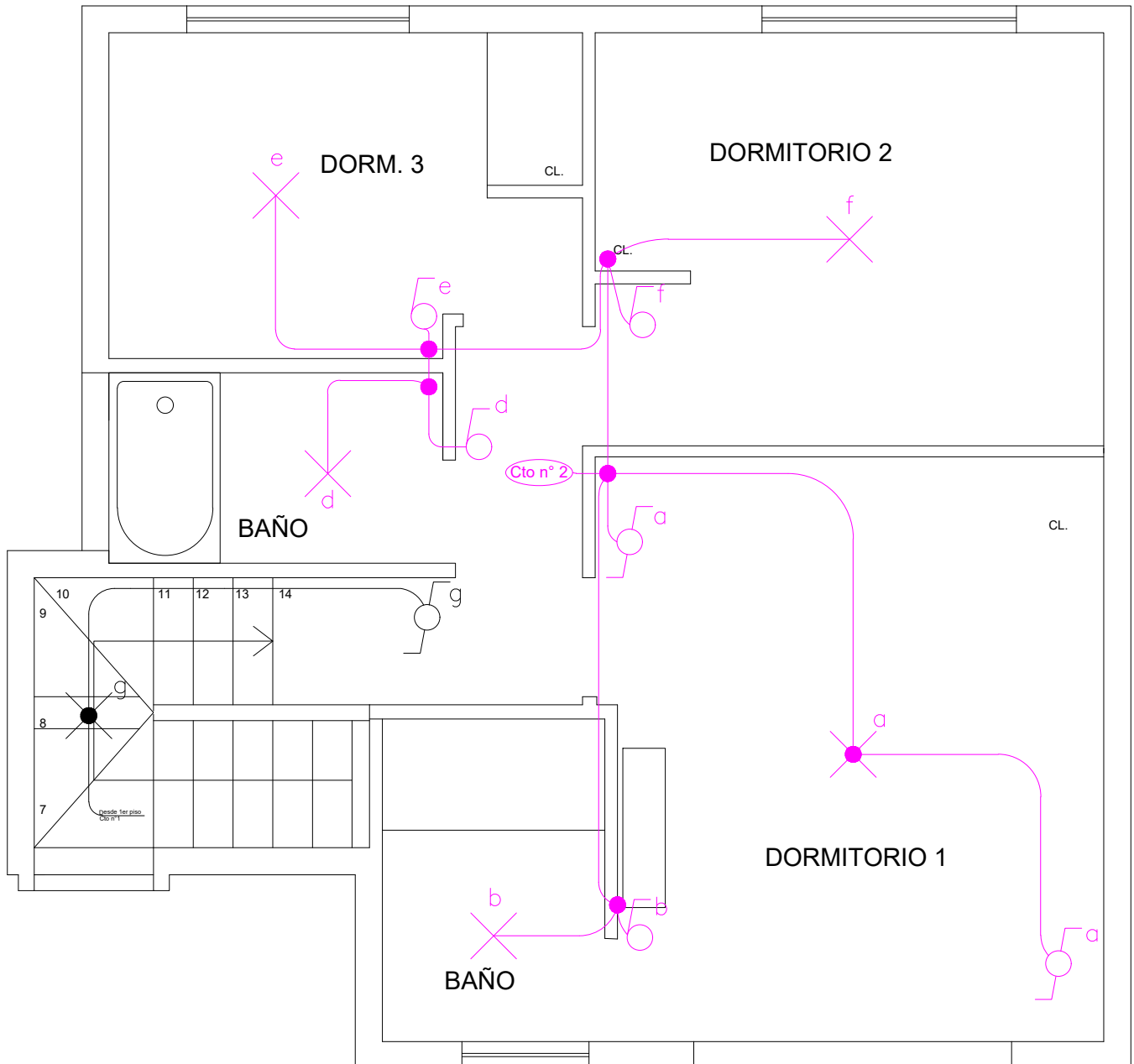
PLANTA ALUMBRADO 2º PISO CASA TIPO AIRE
